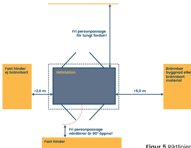
Figur 5 Riktlinjer ovan mark
