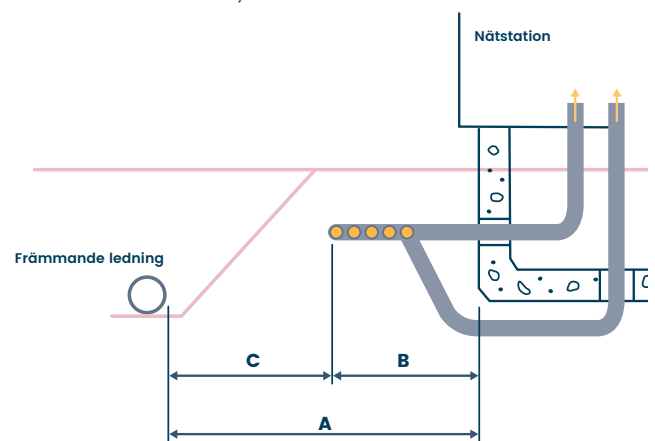
Figur 6 Riktlinjer under mark
